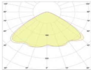
Curva fotométrica 120°
