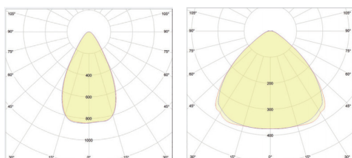
Curva fotométrica 60°
