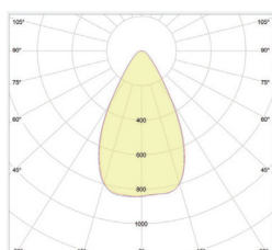
Curva fotométrica 60°
