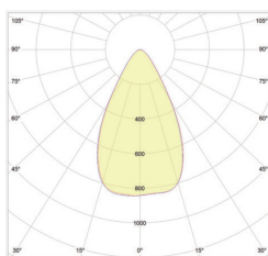
Curva fotométrica 60°
