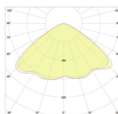
Curva fotométrica 120°
