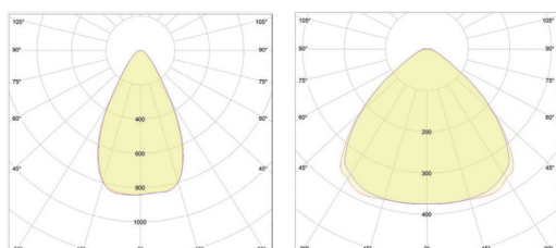
Curva fotométrica 60°
