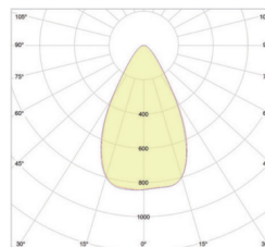
Curva fotométrica 60°
