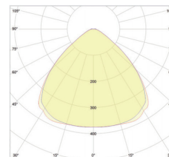
Curva fotométrica 90°
