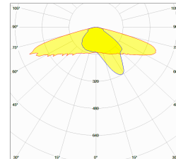
Curva fotométrica TIPO II Médio
